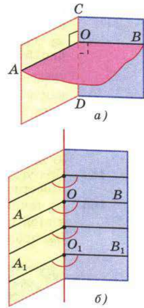
Линейный угол двугранного угла
